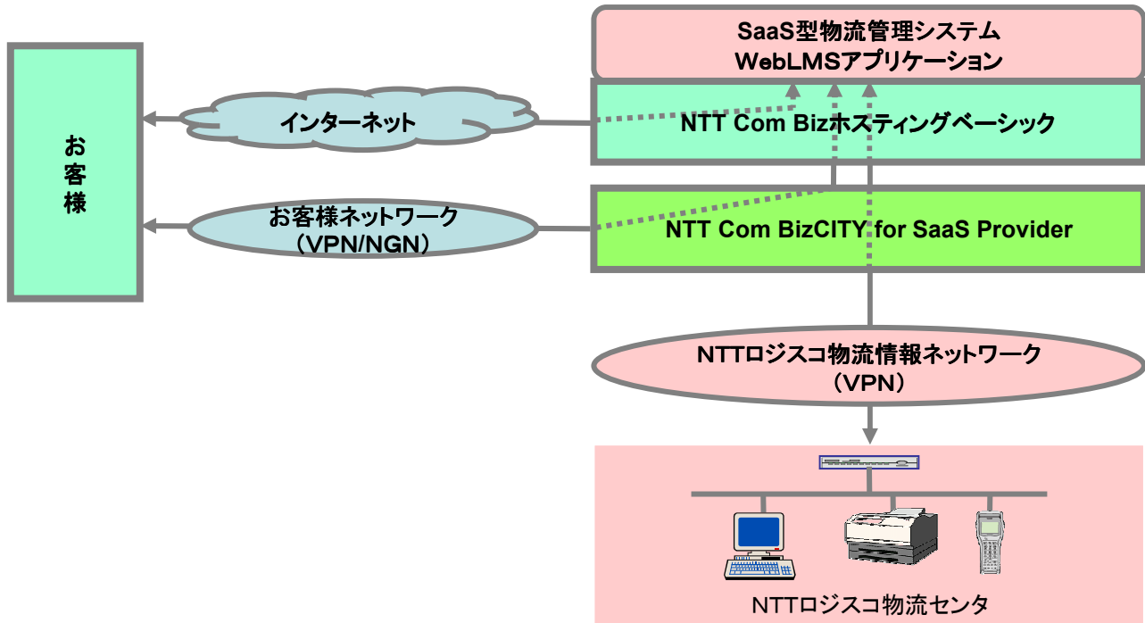
図1 SaaS型Web物流管理システム(WebLMS)の構成
